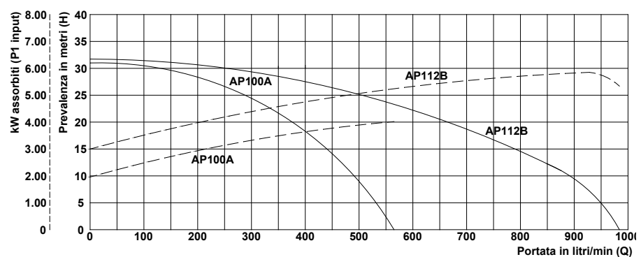
Kurven Hydraulikleistungen (Laufrad offen)
