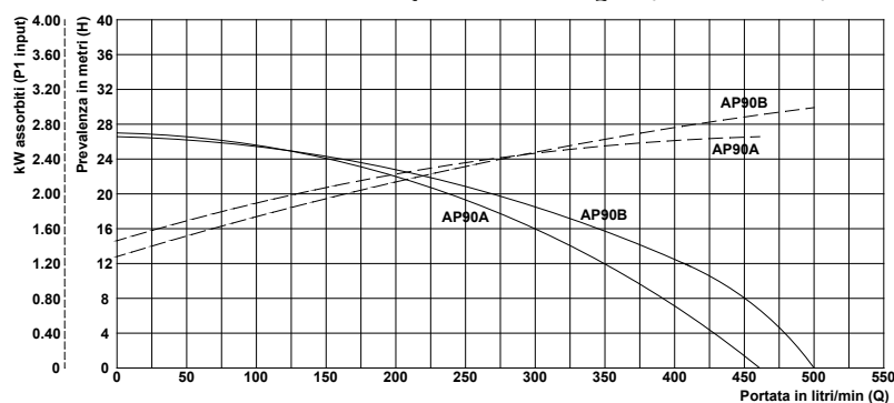
Kurven Hydraulikleistungen (Laufrad offen)
