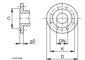
Flanges EN 1092-2
