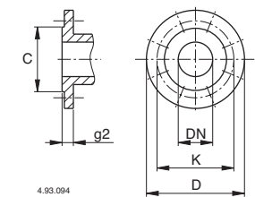
Flanges EN 1092-2
