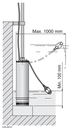
Pumpe stehend
