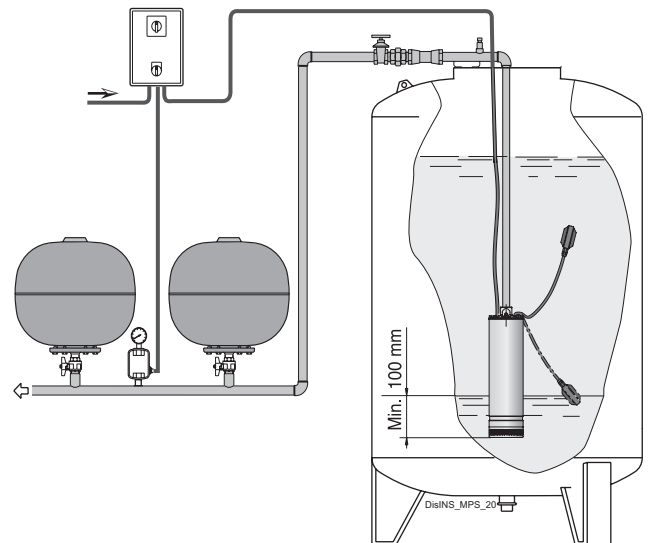
Installationsbeispiele
