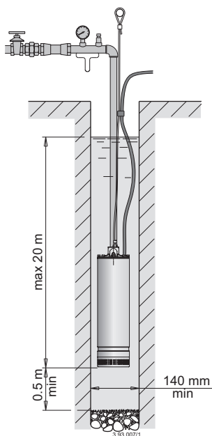
Pumpe aufgehängt
