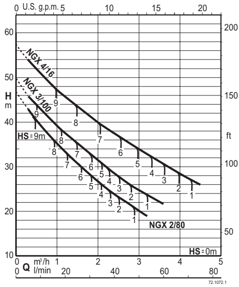
Kennlinien bei verschiedenen Saughöhen
