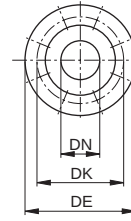
Flanges EN 1092-2
