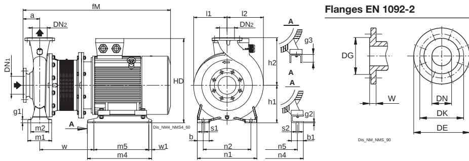
Flanges EN 1092-2
