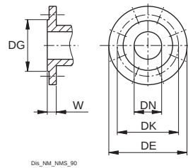
Flanges EN 1092-2
