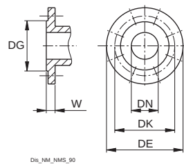
Flanges EN 1092-2
