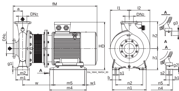
Flanges EN 1092-2
