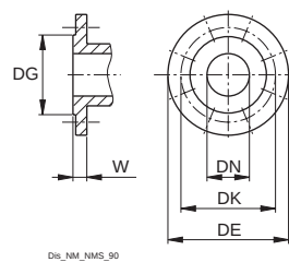
Flansche nach EN 1092-2
