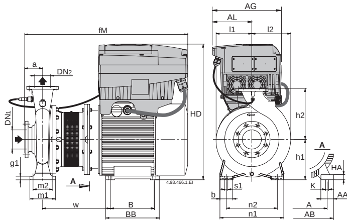
Flansche nach EN 1092-2
