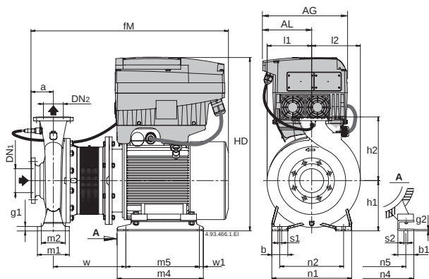
Flansche nach EN 1092-2
