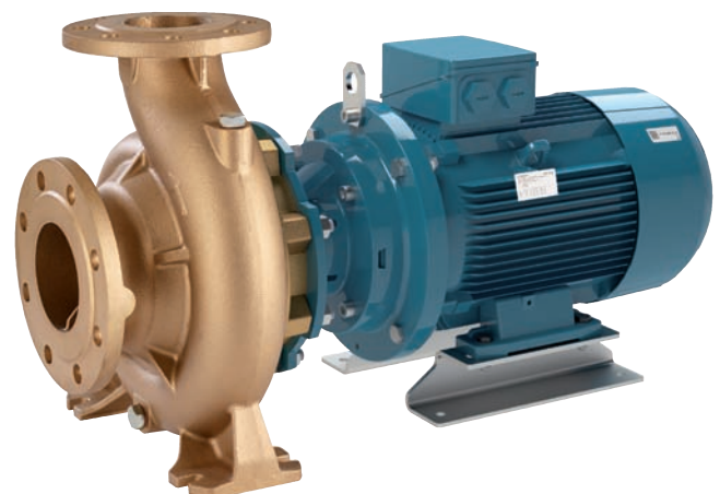
NMS, NMS4 (Ausführung Steckwellenkonstruktion in Grauguss) BNMS, BNMS4 (Ausführung Steckwellenkonstruktion in Bronze)
